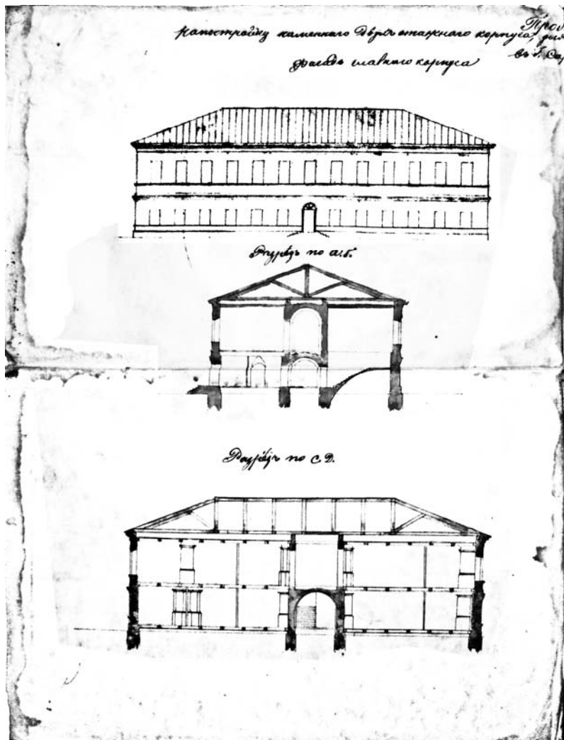
Рис. 3. ГАКО ф.583, оп.492,ед.хр.2. Дело по отношению Сарапульской Уездной земской Управы об утверждении проекта на постройку в Сарапуле больницы. 1869г.
