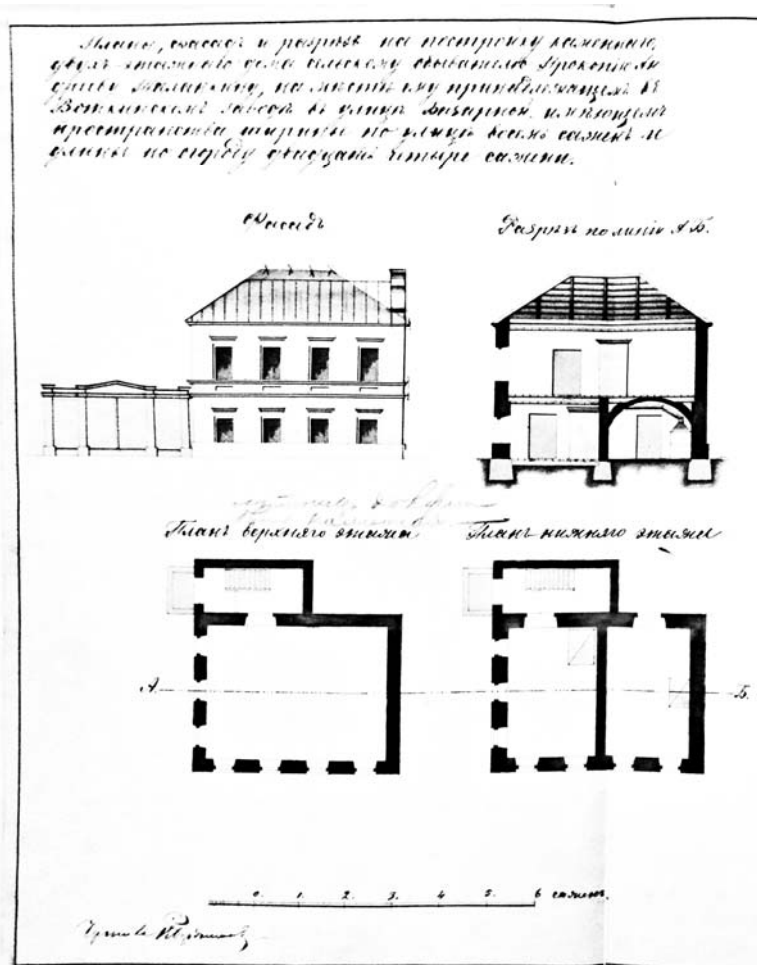
Рис. 38. ГАКО ф.583, оп.494, ед.хр.98. Дело по прошению сельского обывателя Воткинского завода Прокопия Таланкина, об утверждении плана на постройку дома. 1871г.
