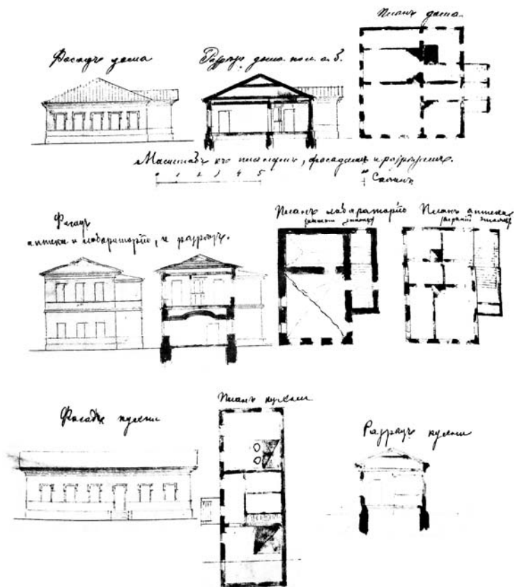
Рис. 5. ГАКО ф.583, оп.492,ед.хр.2. Дело по отношению Сарептурской Уездной земской Управы об утверждении проекта на постройку в Сарепте больницы. 1869г.
