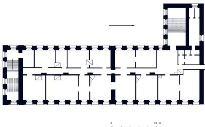
Рис. 18. Дом жилой Дедюхиной. План 2 этажа.
