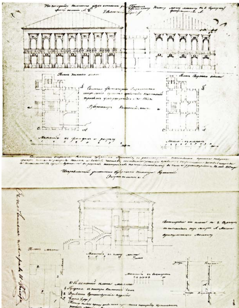
Рис.15. ГАКО ф.583, оп.495, ед.хр.83. Дело по прошению Крестьянина Сарепульского уезда Никона Лукина Мошкина, об утверждении проекта на постройку каменного 2-х этажного дома в городе Сарепуле. 1868г.
