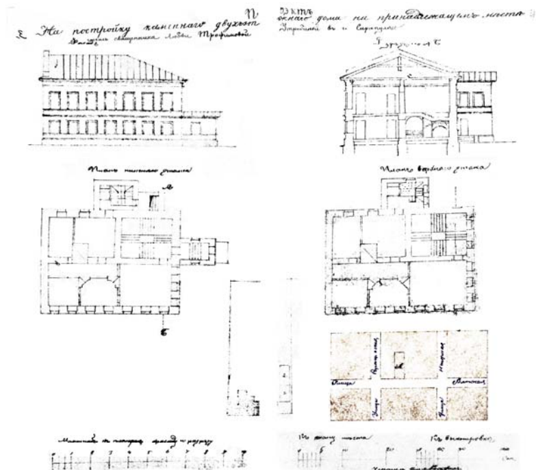
Рис. 21. ГАКО ф.583, оп.491, ед.хр.43. Дело по прошению жены Священника Любови Трофимовны Утробинной, об утверждении проекта на постройку двух - этажного каменного дома в городе Сарепуле. 1868г.
